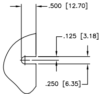
SLOT DETAIL SCALE: 2/1
